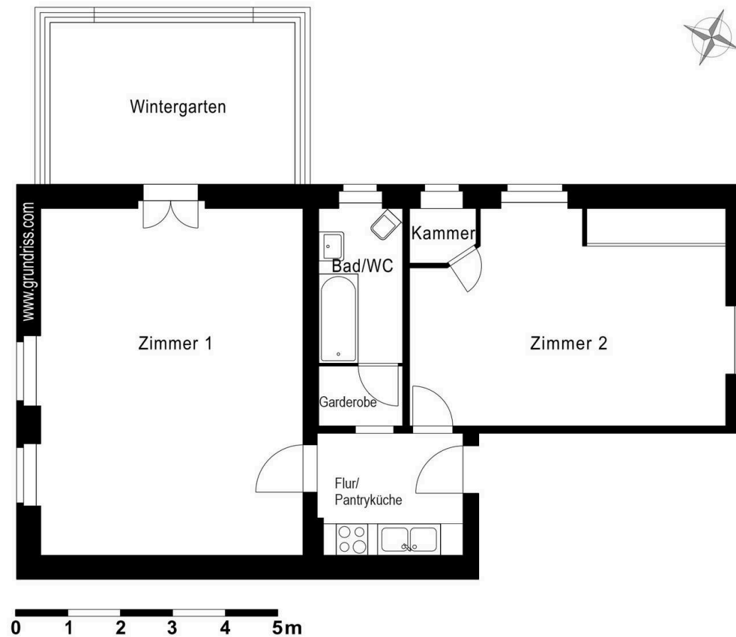
1.Obergeschoss rechts/Wohneinheit Südwest (WE03)
