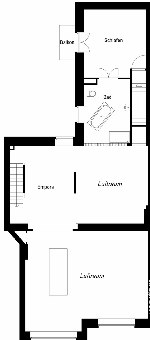
1. Obergeschoss
